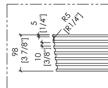
PLINTO A - PLINTH A
